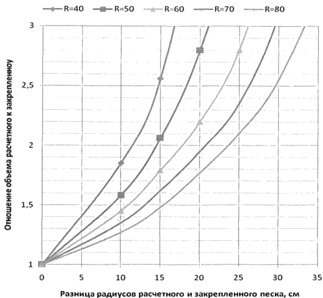
Рисунок У.1 – Отношение расчетного объема песка к закрепленному цементным раствором в зависимости от разницы радиуса расчетного ( R = 40; 50; 60; 70; 80 см) и получаемого закрепленного песка
