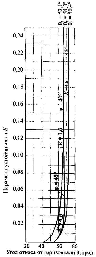
Рисунок В.5 – Графики для определения крутизны откоса при 3 < K \leq 5
