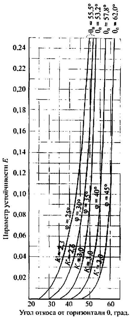
Рисунок В.4 – Графики для определения крутизны откоса при 2 < K < 3
