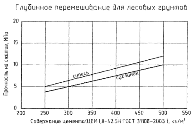
Рисунок Ф.3 – Зависимость прочности грунтоцемента от содержания цемента в 1 м³ ГЦЭ
