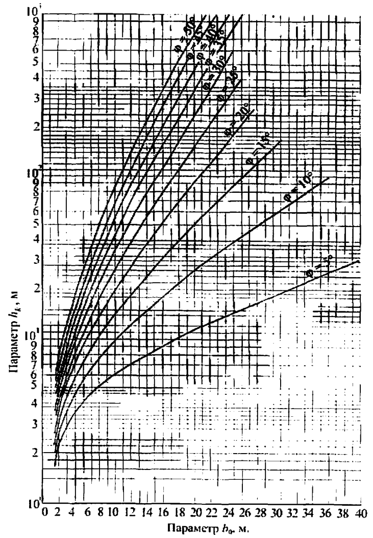
Рисунок В.6 – Графики для определения параметра h_0
